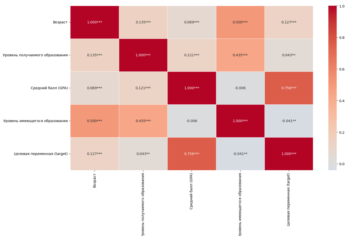
Рисунок 5 – Матрица корреляции числовых признаков и целевой переменной
