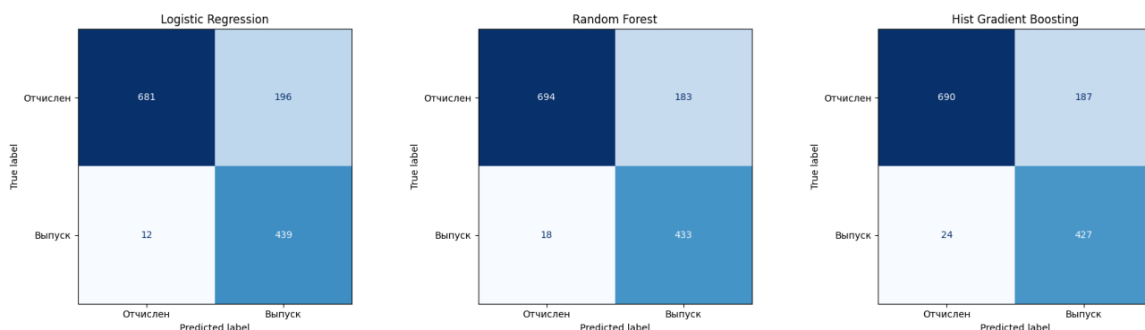
Рисунок 7 – Матрица ошибок
