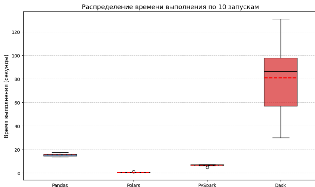
Рисунок 4 – Распределение времени между Pandas, Polars, PySpark и Dask
