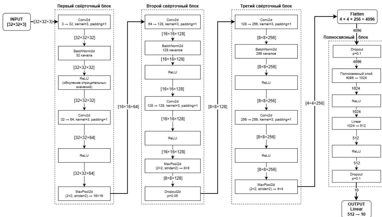
Рисунок 1 – Архитектура модели Oracle (три сверточных блока + полносвязный)
