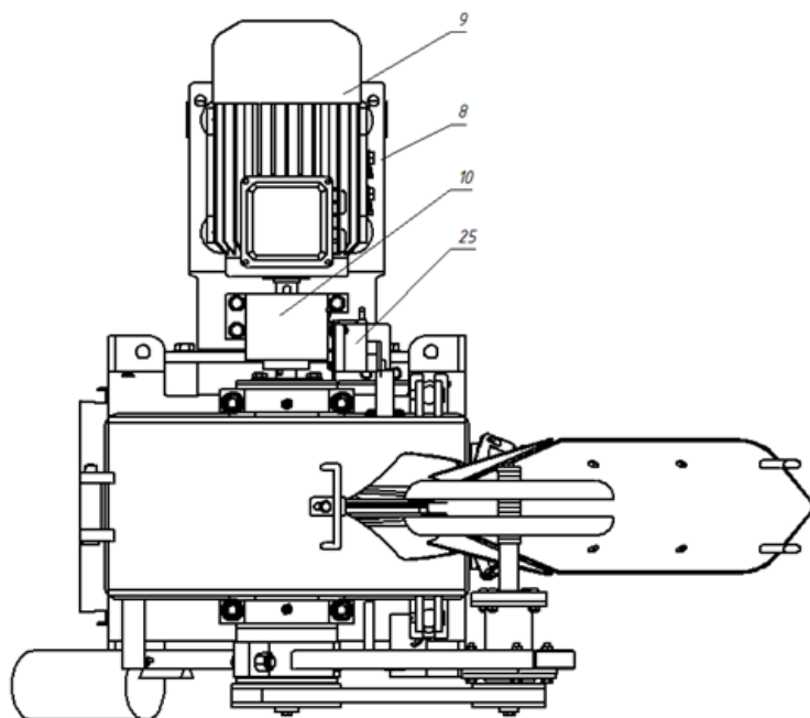
Рисунок 2 – Машина для филетирования рыбы, общий вид сверху
